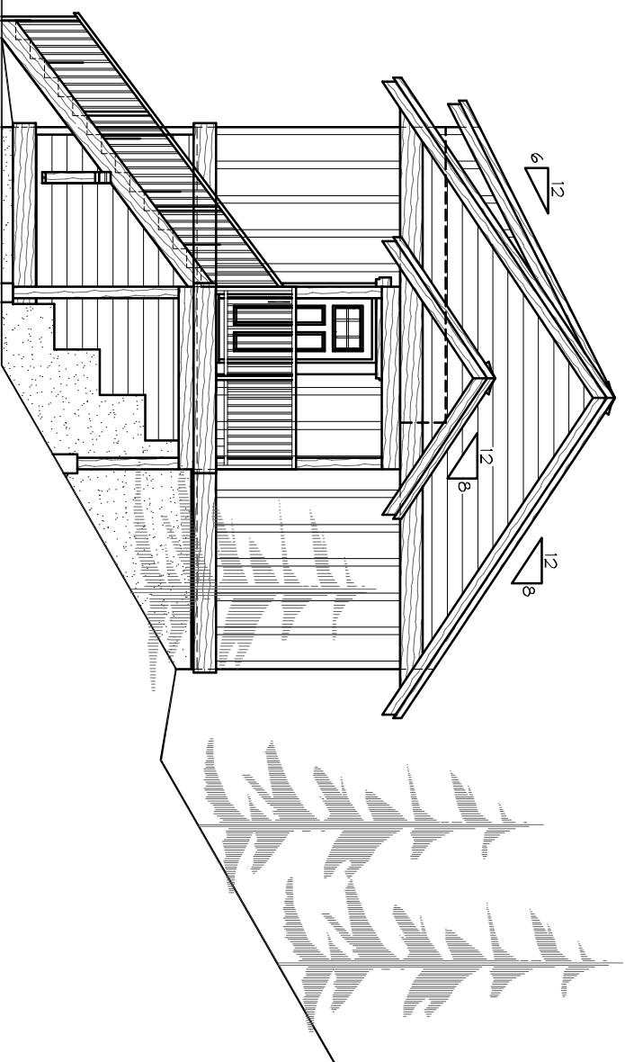
RIGHT ELEVATION
